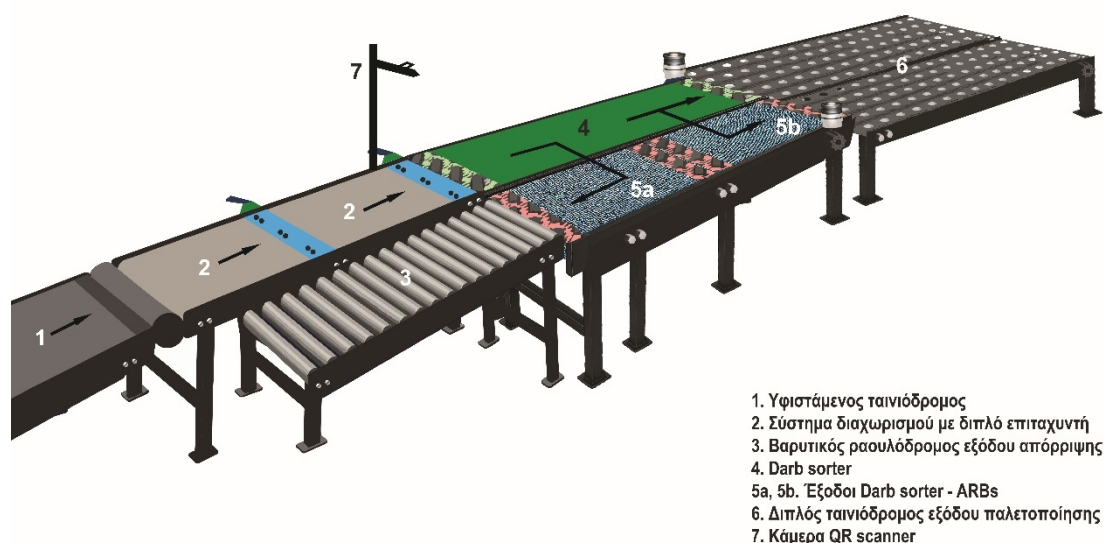
Εικόνα 4: Νέο σύστημα αυτοματισμών
