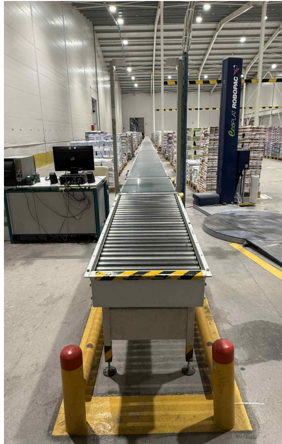
Εικόνα 1: Διάταξη υφιστάμενου ταινιοδρόμου
